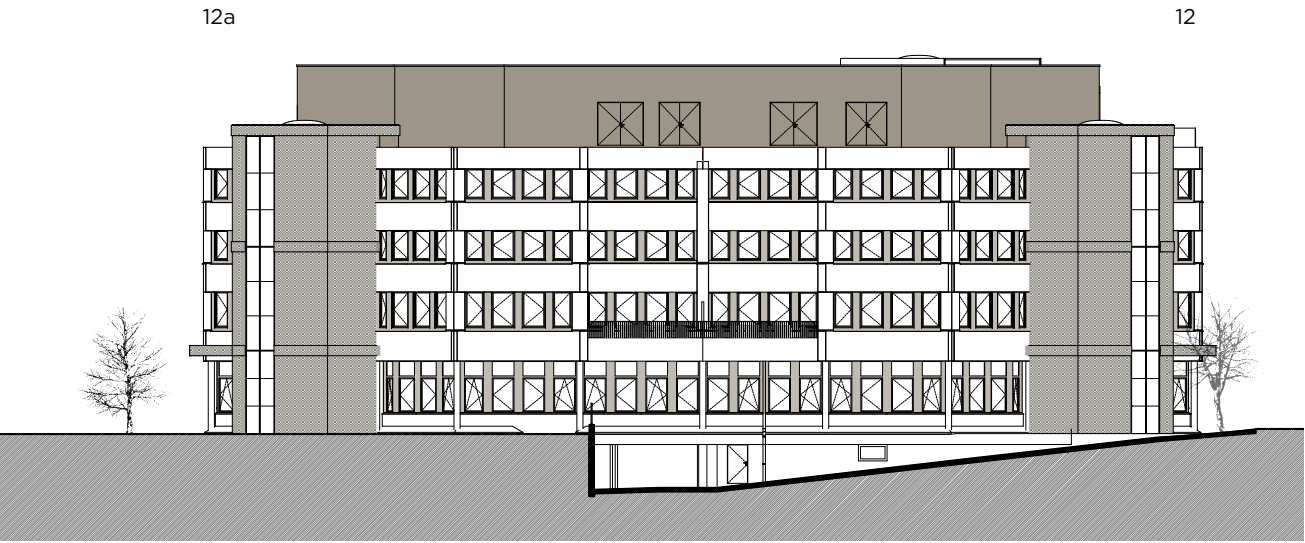
Façade ouest
